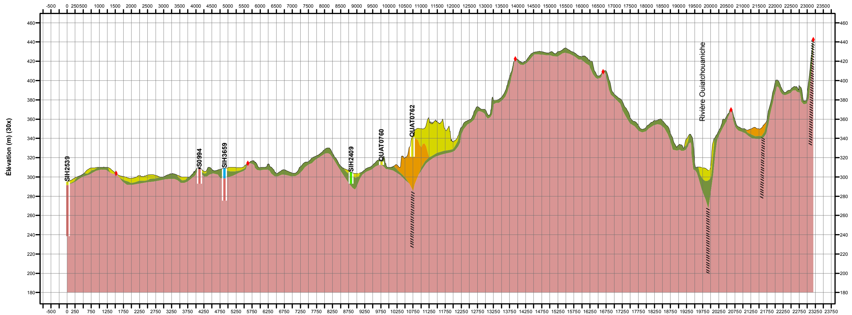
Coupe stratigraphique O-O' - Coupe #15
