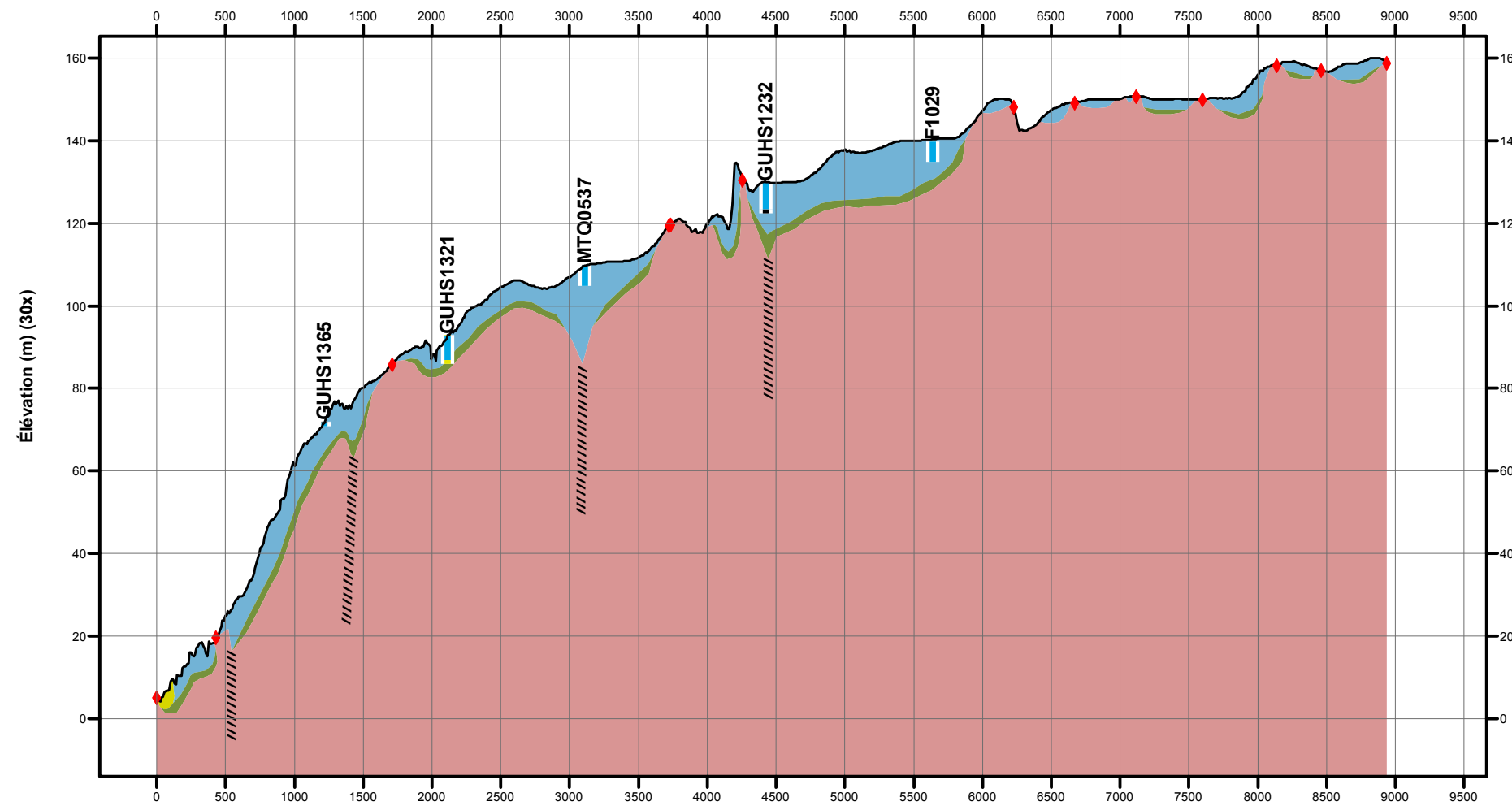
Coupe stratigraphique D-D' - Coupe #12
