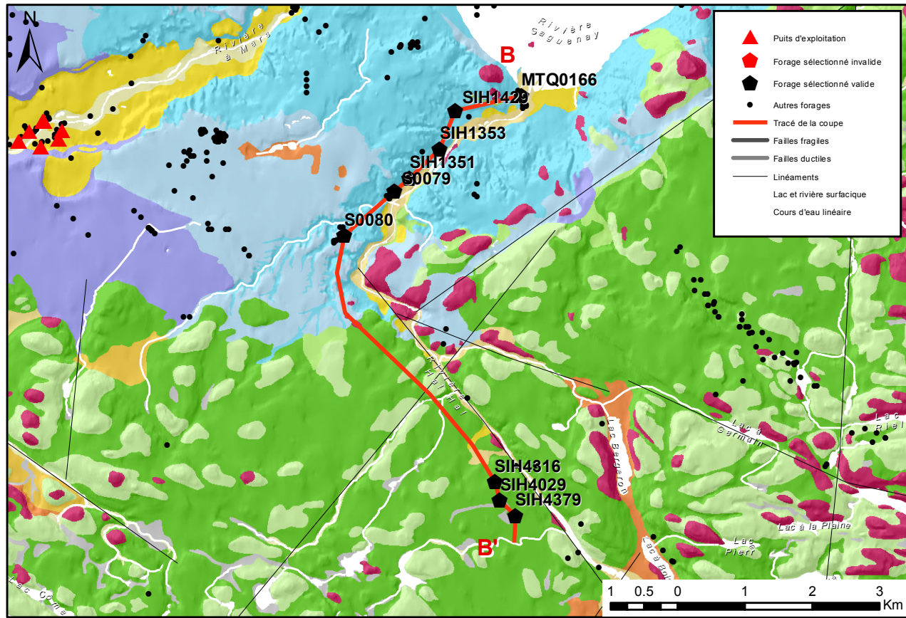
NORD-EST B SUD-OUEST / NORD-OUEST SUD-EST B'
