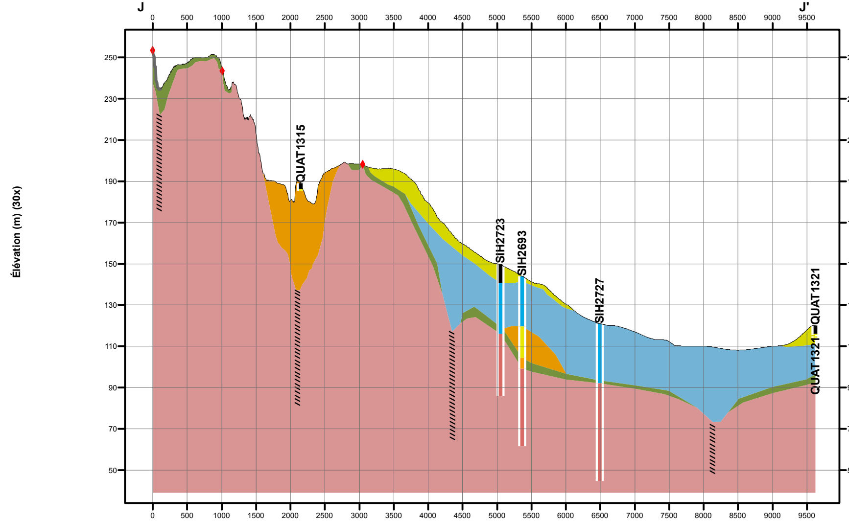
Coupe stratigraphique J-J' - Coupe #10
