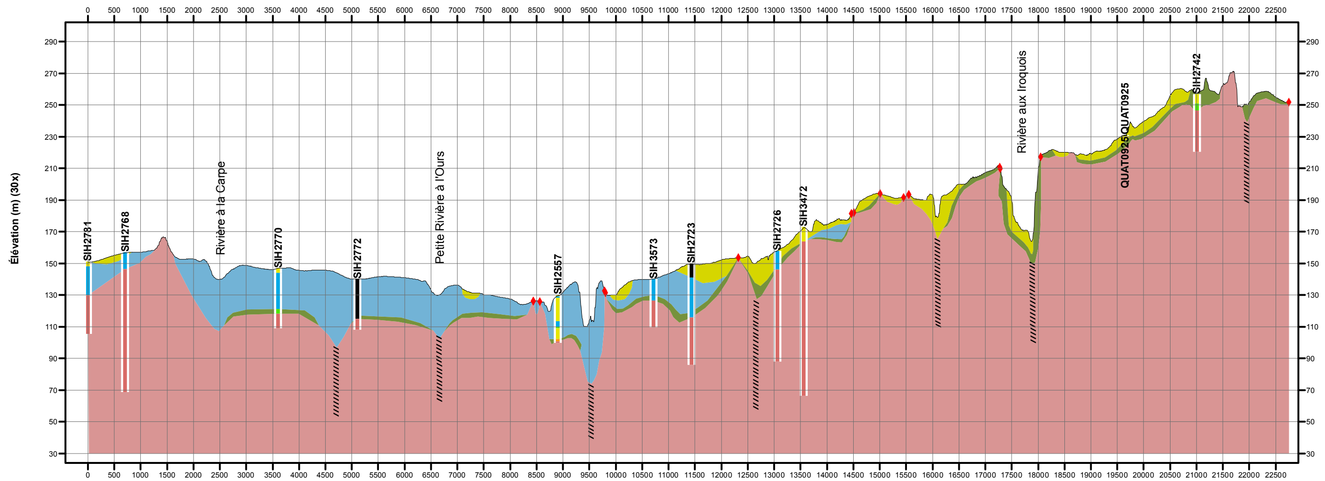
Coupe stratigraphique B-B' - Coupe #3 SAGUENAY-LAC-SAINT-JEAN QUÉBEC
