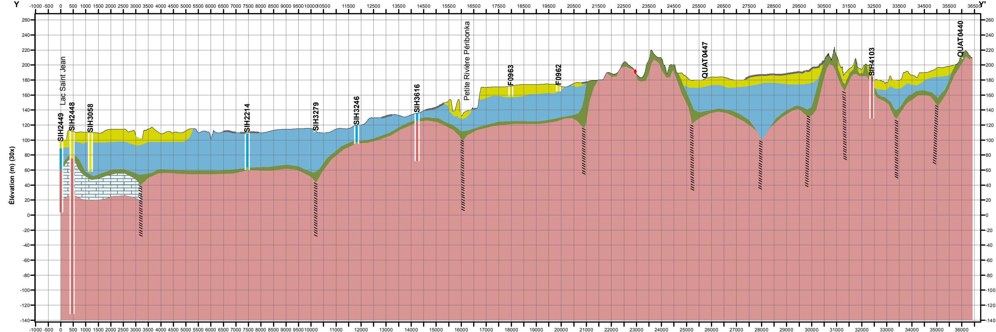
Coupe stratigraphique Y-Y' - Coupe #29
