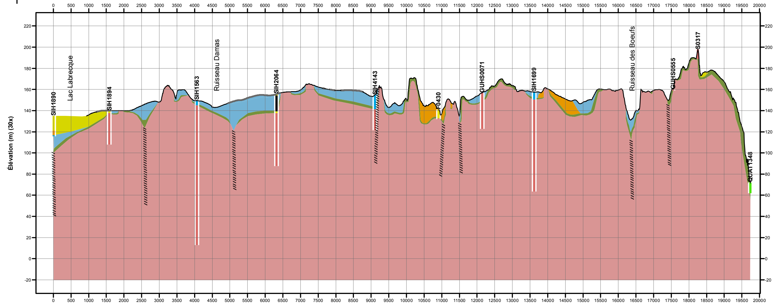
Coupe stratigraphique T-T' - Coupe #27
