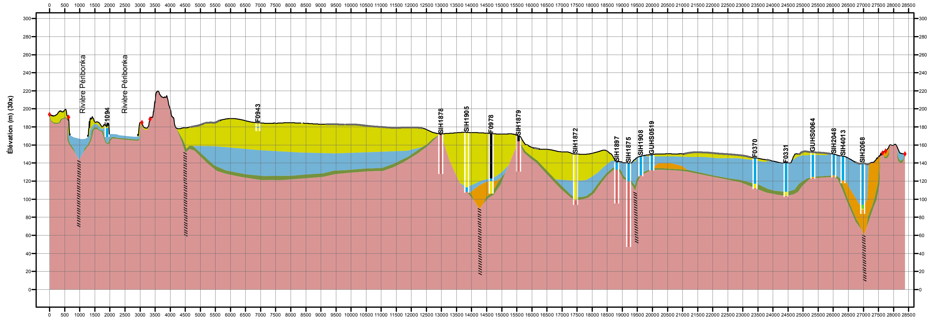
Coupe stratigraphique M-M' - Coupe #19
