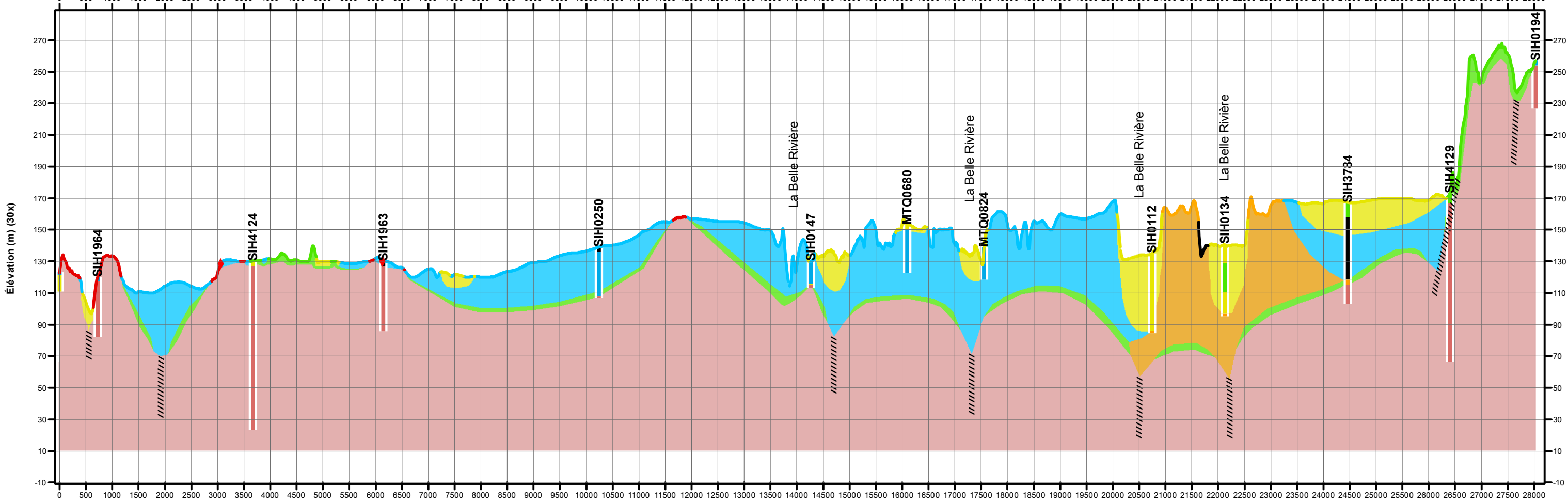
Coupe stratigraphique A-A' Coupe #2 SAGUENAY-LAC-SAINT-JEAN QUÉBEC
